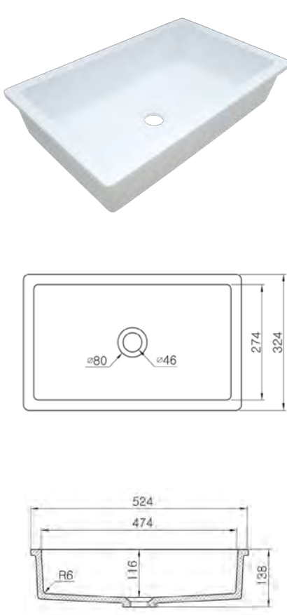
B3190
