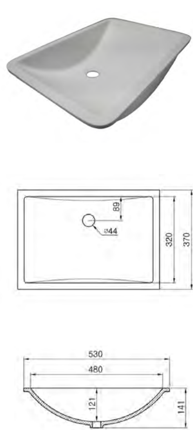
B3192
